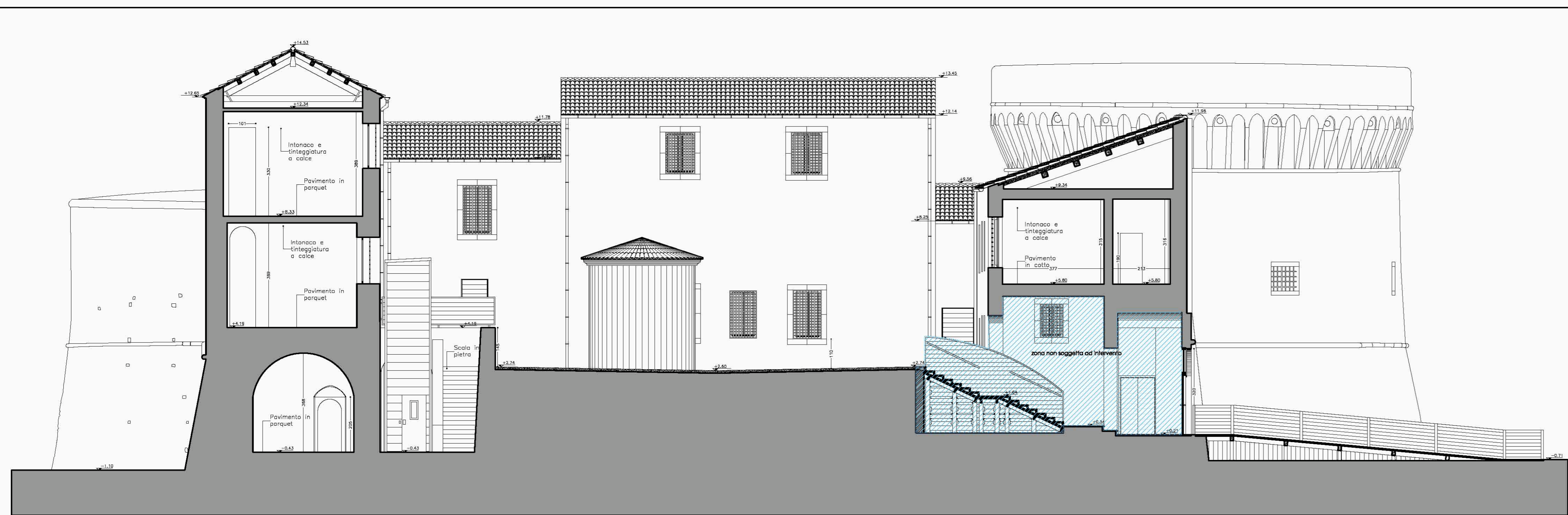
Sezione B-B' Sc. 1:100
