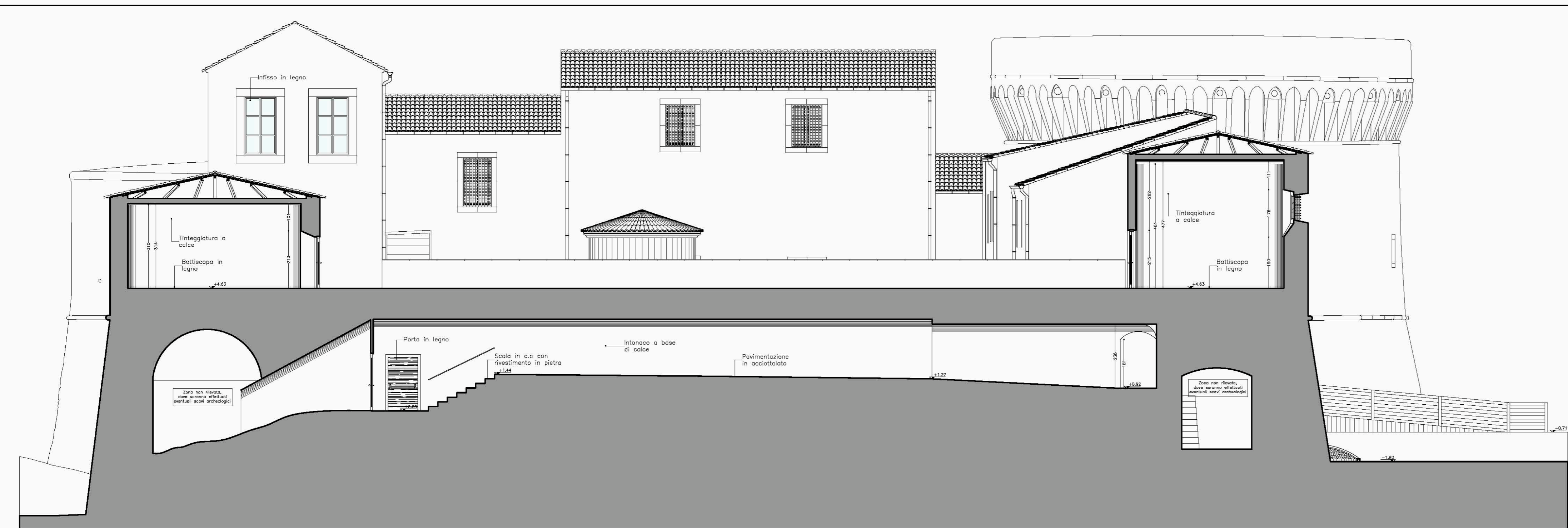
Sezione A-A' Sc. 1:100
